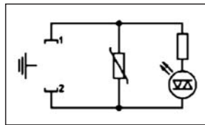
Схема подключения X30, V32
