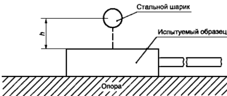
Рисунок F.2 - Испытательная установка
