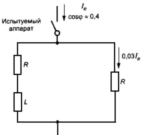
Рисунок С.2 - Упрощенная схема (см. С.3.2.1)
