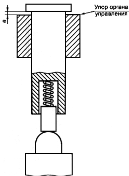
Рисунок 3 - Разность \epsilon между остаточным ходом органа управления и контактного элемента
