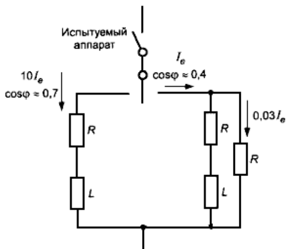
Рисунок С.1 - Полная схема (см. С.3.2.1)
