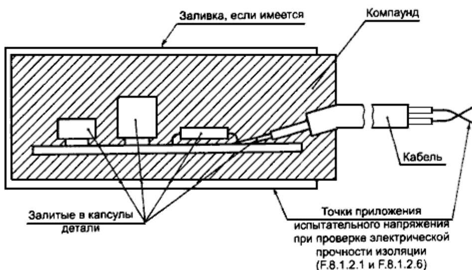
Рисунок F.1 - Изоляция заливкой в капсулы
